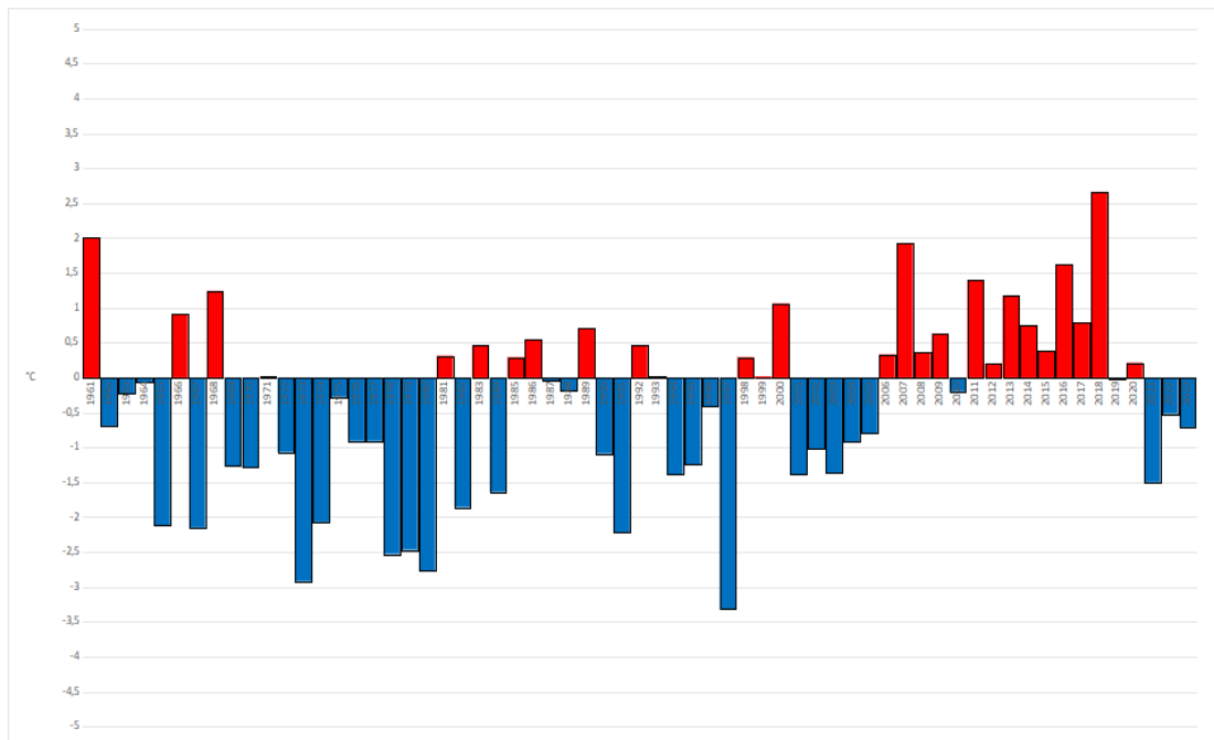
Andamento anomalia della temperatura media regionale del mese di aprile dal 1961 rispetto alla media 1991-2020 (°C). Negli ultimi tre anni, il mese di aprile è stato più freddo della media.
