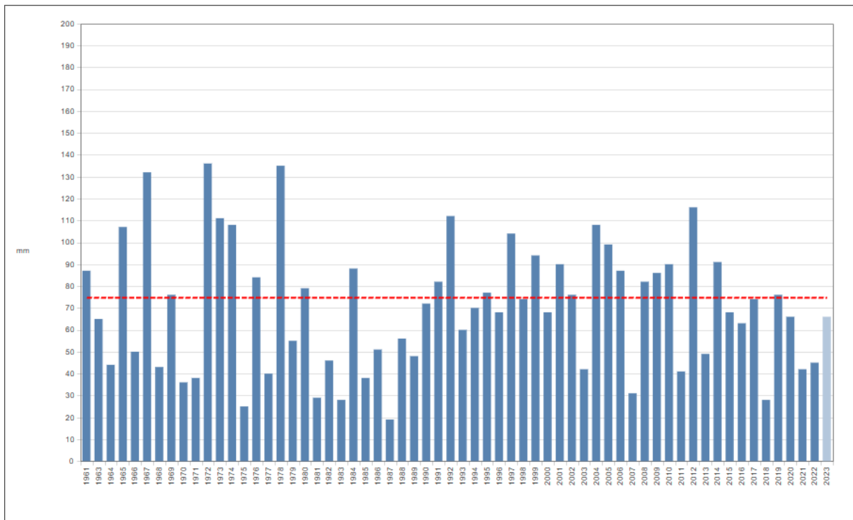
Andamento precipitazione media totale regionale del mese di aprile dal 1961 (mm); la linea tratteggiata rossa rappresenta la media 1991-2020 (mm). Per il quarto anno consecutivo il mese di aprile risulta meno piovoso del normale.
