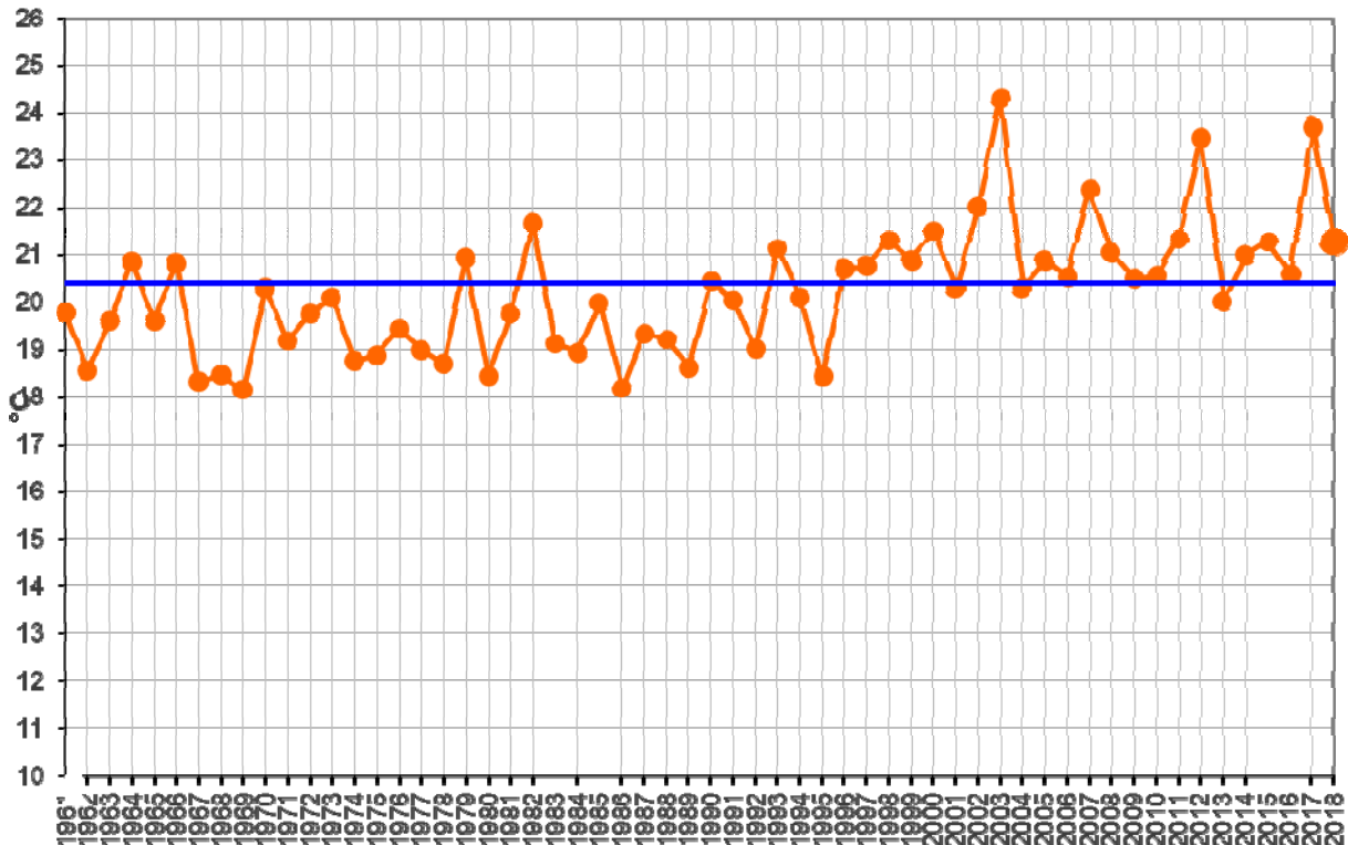
Regione Marche. Andamento temperatura media del mese di giugno dal 1961 (°C); la linea blu rappresenta la media 1981-2010 (°C).
