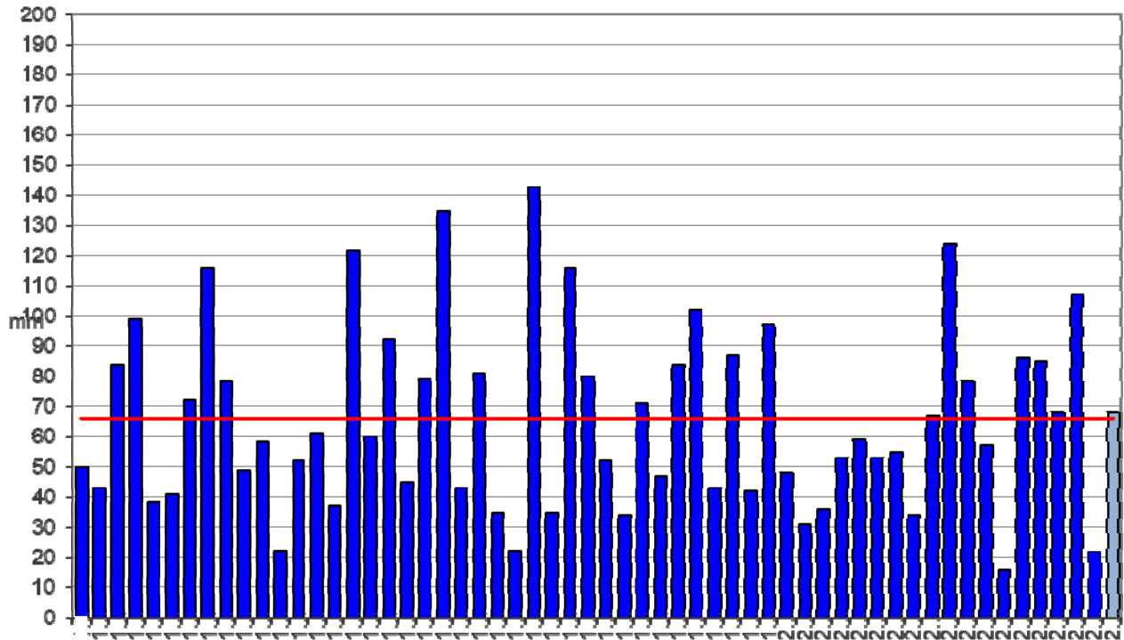
Regione Marche. Andamento precipitazione media del mese di giugno dal 1961 (mm); la linea rossa rappresenta la media 1981-2010 (mm).
